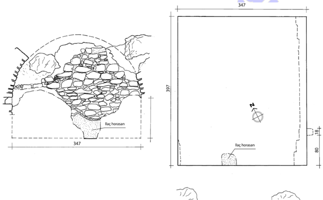
Fig. 34b Plan & prerje e sterës
